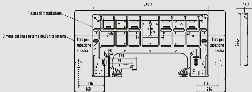
Posizione relativa tra l'unità interna e la piastra di installazione
