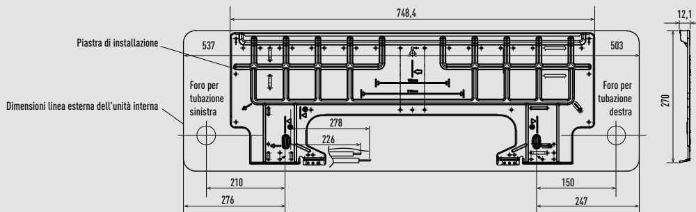
Posizione relativa tra l'unità interna e la piastra di installazione
