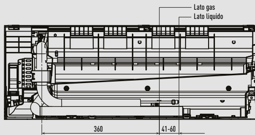
Posizione relativa tra l'unità interna e la piastra di installazione
