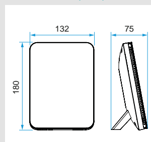
installazione tramite piedistallo
